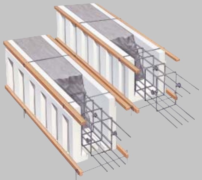
Schematische weergave van het gebruik van de vaste U-vormige (boven) en de samengestelde PS-funderingsbekisting (onder)
